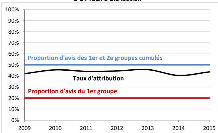
2-2 : Taux d’attribution
